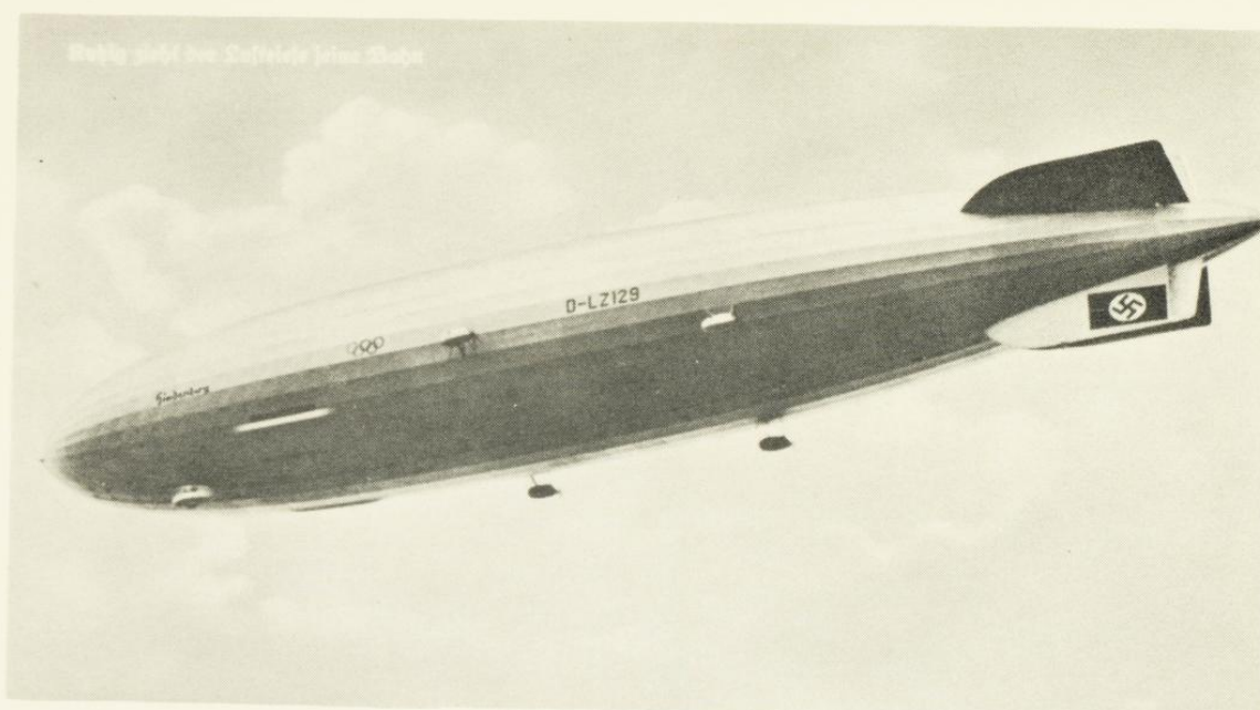
Das neue deutsche Zeppelin-Luftschiff L. Z. 129 Das größte Luftschiff der Welt. Länge 248 m. Höhe 44,7 m, größter Durchmesser 41,2 m. Vortriebsmaschinen: 4 Mercedes-Benz Dieselmotore von je 1100 PS Geschwindigkeit von etwa 130 Stdkm.
